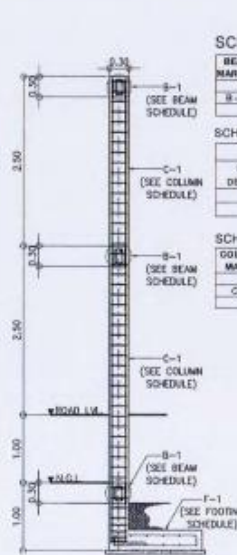
COLUMN SECTION SCALE: 1:400
