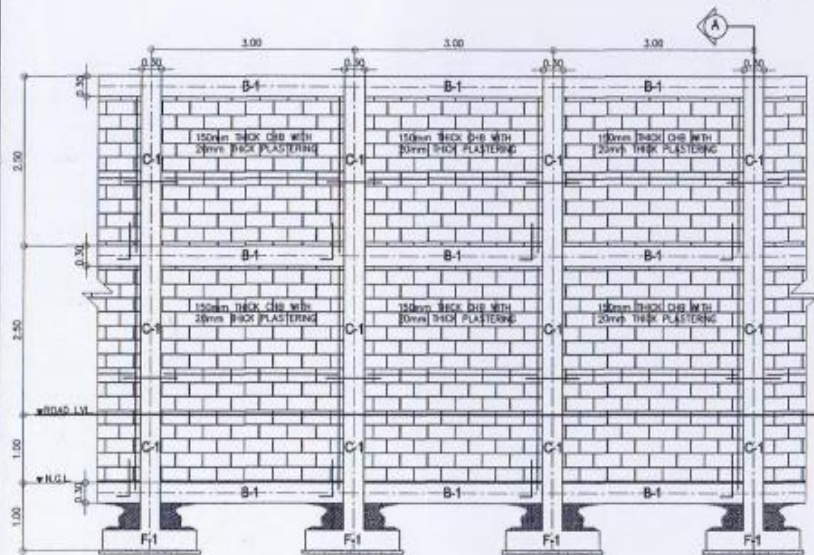
WALL ELEVATION SCALE: 1:400
