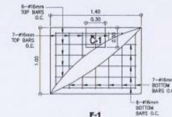
FOOTING DETAIL SCALE: 1:200
